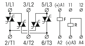
fig. 1. Wiring diagram
