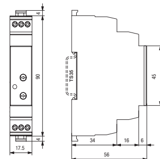
fig. 4. dimensions (mm)
